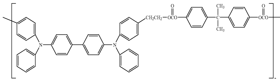
TPD-PMAA
