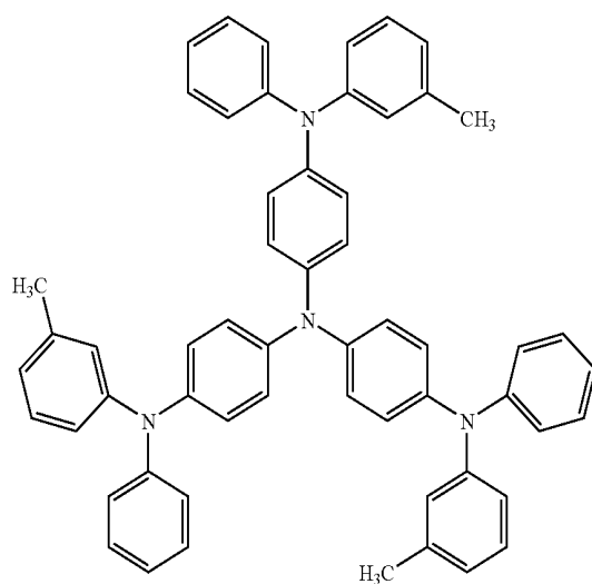
m-MTDATA
