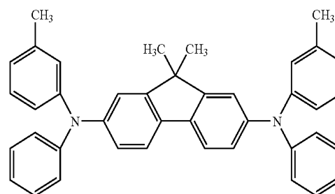
DTDPL
