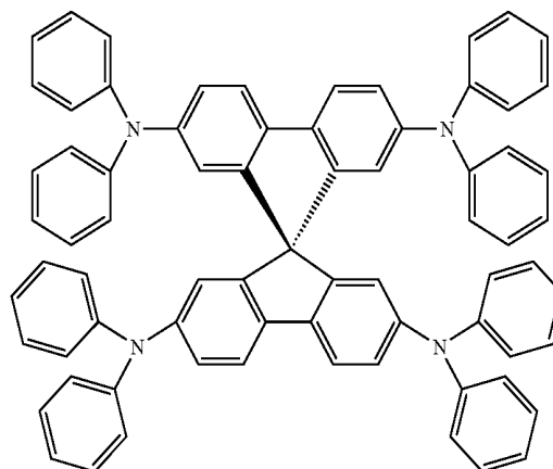
DTDPL
