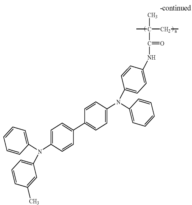
TPD-PMAA
