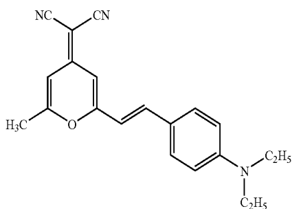
DCM-1
