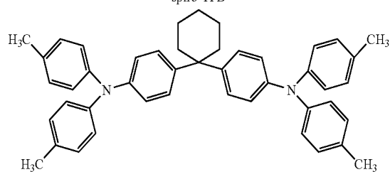
TPAC
